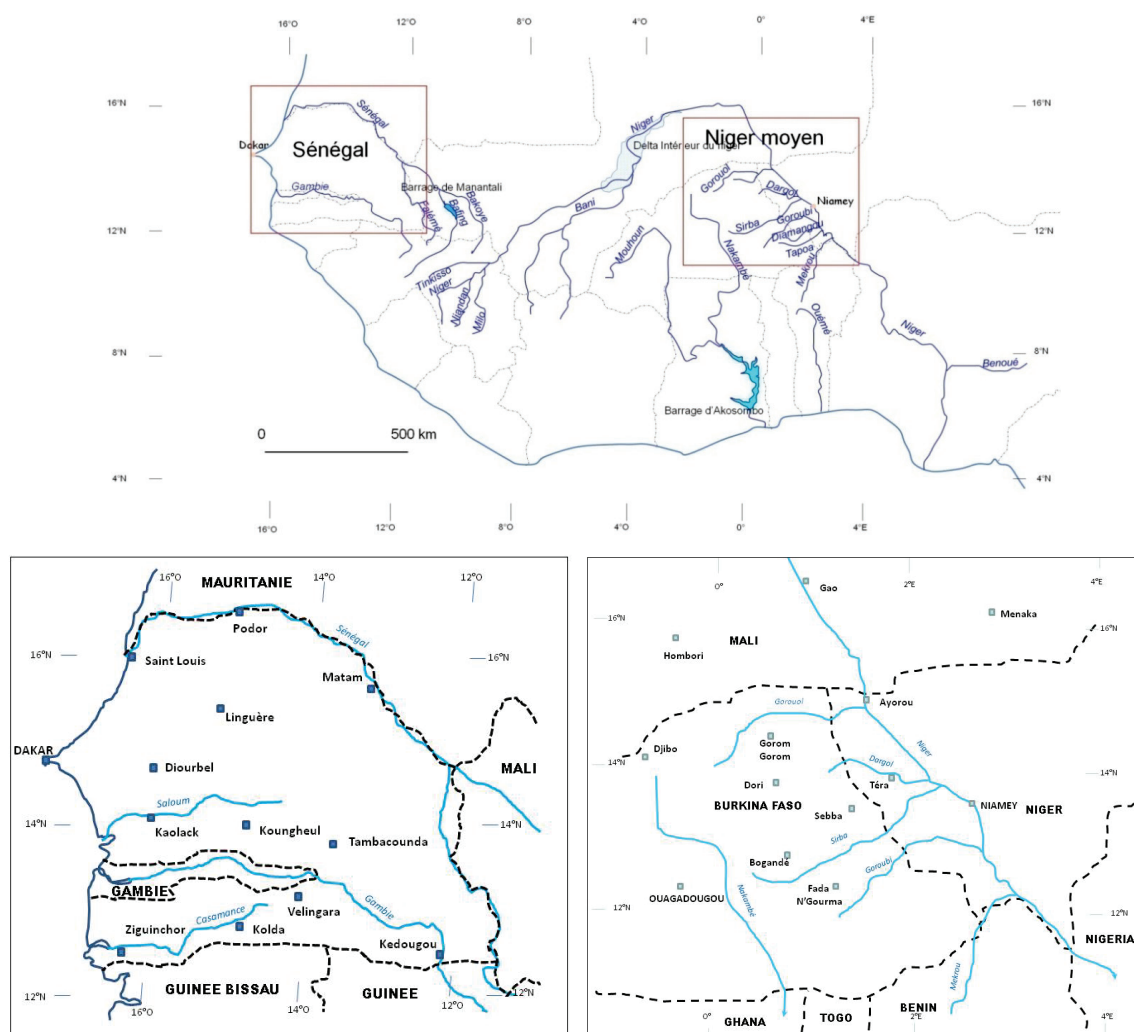
Figure 2 : Localisation (en haut) des deux sous-régions (Sénégambie et bassin du Niger Moyen) où la pluviométrie est analysée, ainsi que des 12 postes pluviométriques utilisés respectivement dans cette étude pour la Sénégambie (en bas à gauche) et pour le bassin du Niger Moyen (en bas à droite). Location of the two areas (Senegambia and Middle Niger River Basin) analyzed in rainfall, and location of the rain gauges used for the analyze in both areas: Senegambia (left) and Mid Niger Basin (right).
