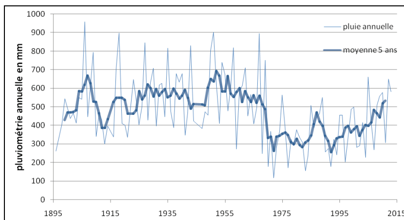
Figure 5 : Evolution de la pluviométrie annuelle à Dakar de 1895 à 2013, avec la présence d'une rupture nette de stationnarité après 1968. Annual rainfall evolution at Dakar station from 1895 to 2013: a remarkable break occurred after 1968.
