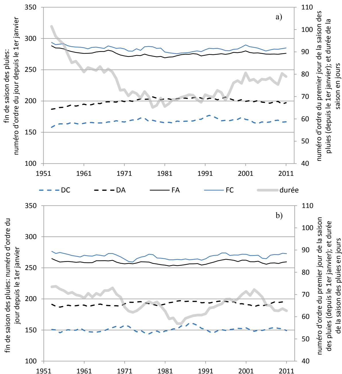
Figure 9 : Date de début et de fin climatique et agronomique, ainsi que la durée de la saison des pluies entre 1951 et 2013 : a) en Sénégambie ; b) dans le bassin du Niger Moyen (DC = début climatique ; DA = début agronomique ; FA = fin agronomique ; FC = fin climatique). Date of climatic and agronomic beginning, end and duration of rainy season from 1951 to 2013. a) in Senegambia; b) in the Middle Niger River Basin; (DC: climatic beginning ; DA: agronomic onset; FA : agronomic end; FC: climatic end).
