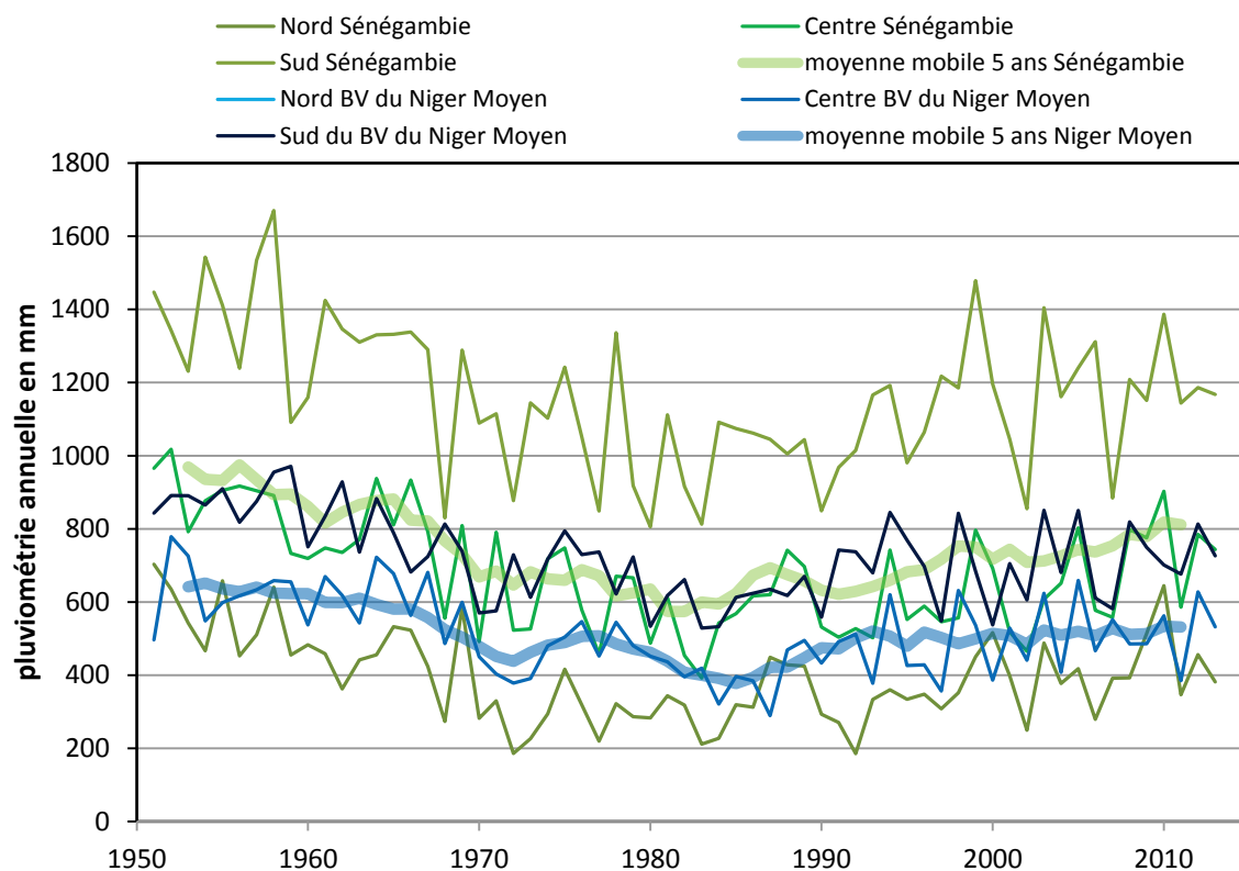
Figure 4 : Evolution de la pluviométrie annuelle moyenne en Sénégambie et dans le Bassin du Niger Moyen de 1951 à 2013. Mean annual rainfall evolution in Senegambia and the Middle Niger River Basin from 1951 to 2013.
