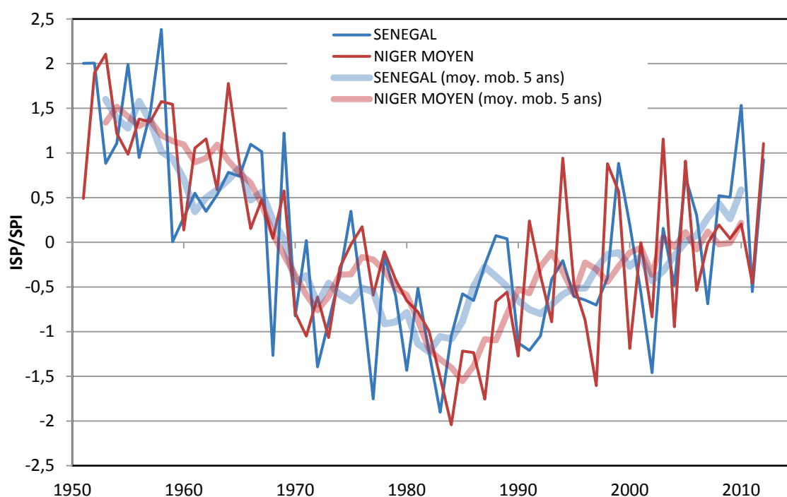
Figure 3 : Evolution de 1951 à 2013 de l'indice pluviométrique (ISP : Indice Standardisé des Précipitations) et de sa moyenne mobile sur 5 ans pour la Sénégal et le bassin du Niger Moyen. 1951-2013 period trends of the SPI (Standard Precipitation Index) and its 5-years mobile average (Standard Precipitation Index) for Senegambia and the Middle Niger River Basin.
