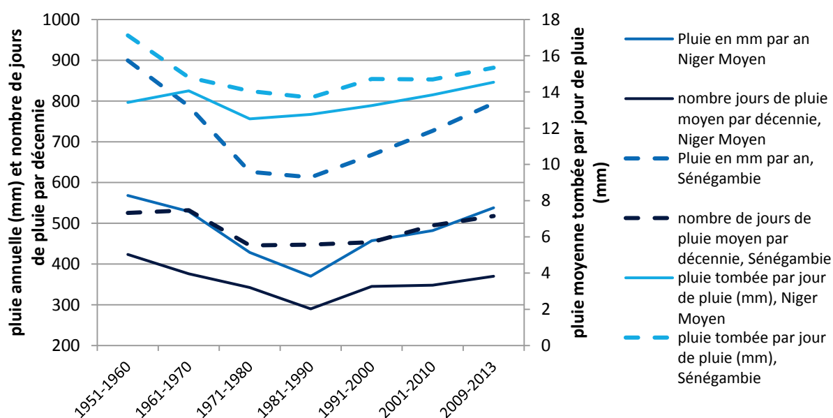
Figure 6 : Evolution décennale de la pluie, du nombre de jours de pluie et de la hauteur moyenne tombée par jour de pluie au Sénégal et dans le Bassin du Niger Moyen (calculés sur la période 1951-2013) ; la dernière période prise en compte est de 5 ans (2009-2013). Decennial evolution of rainfall, yearly number of rainy days, and mean daily rainfall per rainy day in Senegambia and in the Middle Niger River Basin; the last period is a 5-years one 2009-2013.
