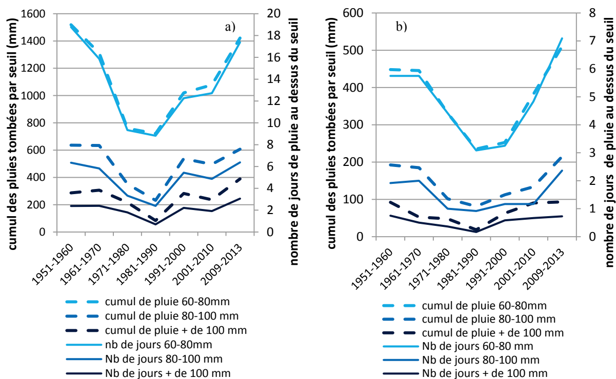
Figure 8 : Evolution des précipitations de fort cumul en 24 heures en Ségambie (a) et dans le bassin du Niger Moyen (b) : nombre de jours de précipitations supérieures à 60, 80 et 100 mm en moyenne annuelle et cumul de pluie apporté par ces jours de pluie intense (valeur absolue par décennie, arbitrairement multipliée par deux pour la période de cinq ans 2009-2013). Evolution of high daily precipitation events in Senegambia (a) and in the Middle Niger River Basin (b): number of days with rainfall higher than 60, 80 and 100 mm in 24h (annual mean), and cumulated rainfall for these intense rainy days (total per decade, X 2 for the 2009-2013 5-years period).
