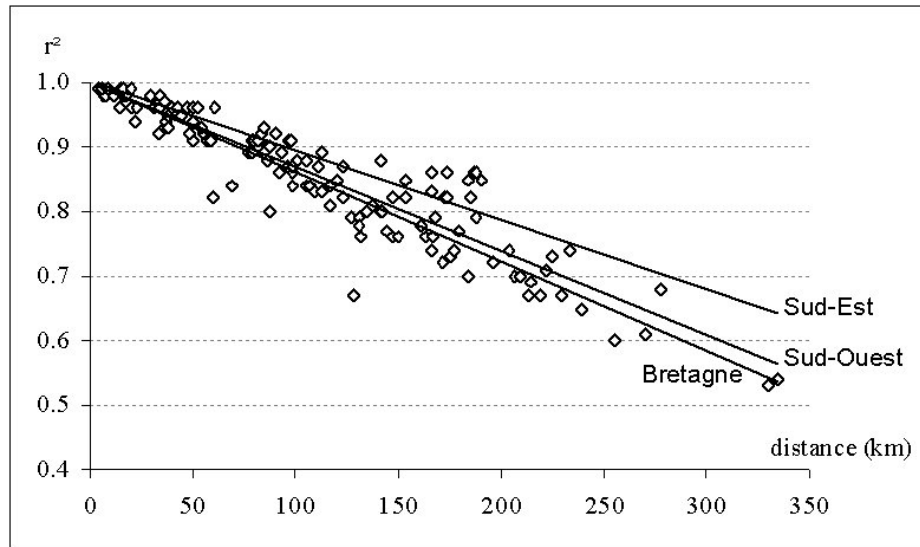
Figure 2 : Coefficients de corrélation des valeurs de rayonnement global entre deux points de mesures en fonction de leur distance. Radiation correlation coefficients between 2 stations as a function of the distance.
