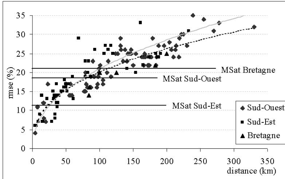
Figure 4 : Extrapolation du rayonnement global et distance critique. Extrapolation of global radiation and critical distance.
