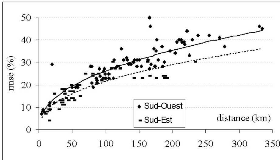
Figure 5 : Performance de la reconstitution du rayonnement par substitution des postes entre eux. Results of the reconstitution of the global radiation by substitution of stations.
