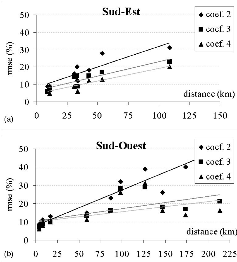
Figure 6. Reconstitution par utilisation de la structure spatiale de MétéoSat (a : Sud-Est, b : Sud-Ouest) en fonction des indices de disponibilité. Reconstitution of global radiation using spatial structure of MeteoSat (a: South-East, b : South-West) according to the reliability coefficients.
