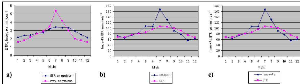
Figure 3 : Valeurs mensuelles moyennes de l'évapotranspiration réelle calculées sur la période du 1 er janvier 2005 au 31 décembre 2010 et valeurs mensuelles moyennes de l'irrigation de l'orangerie de la station d'étude (valeurs constantes sur la période du 1 er juin 2005 au 26 avril 2013) : a) comparaison de l' ETR_{calculée} avec l'irrigation ( ETR vs I_{moy} ) ; b) comparaison de l' ETR_{calculée} avec l'irrigation à laquelle on ajoute les précipitations incidentes ( P_i ) ( ETR vs I_{moy}+P_i ) ; c) comparaison de l' ETR_{calculée} avec l'irrigation à laquelle on ajoute les précipitations au sol P_s (soit P_i-I_n ) ( ETR vs I_{moy}+P_s ). Simulated average monthly values of the actual evapotranspiration and the average monthly values of the irrigation of the orange grove of the studies plot over the period of January 1 2005 to December 31 2010 (constant values over the period of June 1 2005 to April 26 2013): a) comparison between Ea_{simulated} and irrigation ( Ea vs I_{mean} ); b) comparison between Ea_{simulated} and irrigation with gross precipitations ( P_i ) ( Ea vs I_{mean}+P_i ); c) comparison between Ea_{simulated} and irrigation with throughfall, P_s ( P_s =gross precipitations-net interception) ( Ea vs I_{mean}+P_s ).
