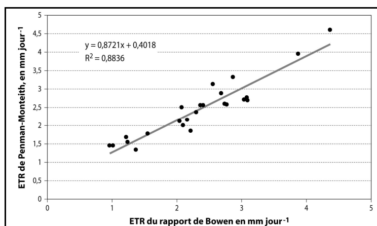
Figure 5 : Relation entre l'évapotranspiration réelle de la savane à Loudetia arundinacea issue de l'équation de Penman-Monteith et du rapport de Bowen ; valeurs journalières lors de la période du 18 septembre au 11 octobre 1998. Relationship between the actual evapotranspiration of savannah with Loudetia arundinacea obtained from Penman-Monteith and Bowen-ratio method; daily values during the period from September 18 to October 11, 1998.
