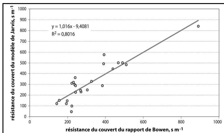
Figure 3 : Relation entre la résistance du couvert de la savane à Loudetia arundinacea issue du modèle de Jarvis-Stewart (Founa-Toutou, 2000) et du rapport de Bowen ; valeurs journalières lors de la période du 18 septembre au 11 octobre 1998. Relationship between the canopy resistance of savannah with Loudetia arundinacea obtained from Jarvis-Stewart model (Founa-Toutou, 2000) and from Bowen-ratio method; daily values during the period from September 18 to October 11, 1998.
