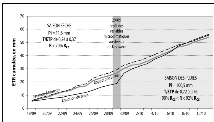
Figure 4 : Evapotranspiration réelle de la savane à Loudetia arundinacea ; valeurs cumulées obtenues par les méthodes de l'équation du bilan, de l'équation de Penman-Monteith et du rapport de Bowen, sur la période du 18 septembre au 11 octobre 1998. Actual evapotranspiration of savannah with Loudetia arundinacea ; cumulated values obtained from the soil-water balance equation, Penman-Monteith equation and Bowen-ratio method, during the period from September 18 to October 11, 1998.
