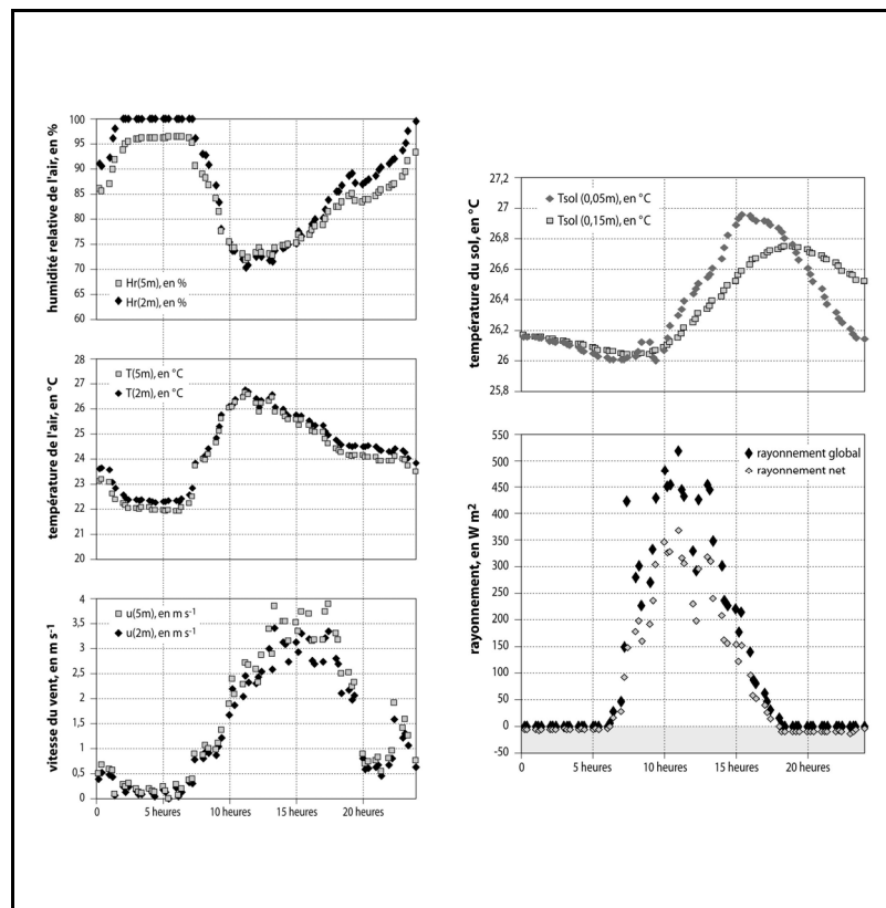
Figure 1 : Evolution au cours de la journée du 29 septembre 1998 (à gauche) de la température moyenne de l'air ( T_{air} ), de l'humidité relative de l'air ( H_r ), de la vitesse du vent ( u ) à 2,0 et 5,0 m au-dessus de la surface du sol de la savane ; (à droite) de la température du sol à 0,05 et 0,15 m de profondeur, du rayonnement global ( R_g ) et rayonnement net ( R_n ) à 6,0 m au dessus de la surface du sol de la savane. Evolution during the day of September 29, 1998 (a) of the mean air temperature ( T_{air} ), relative humidity ( H_r ), wind speed ( u ) 2.0 and 5.0 m above the soil surface of the savannah; (b) mean soil temperature at a depth of 0.05 m and 0.15 m; of global ( R_g ) and net radiation ( R_n ) at 6.0 m above the soil surface of the savannah.
