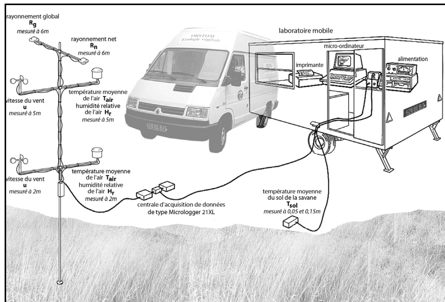
Figure 2 : Schéma du dispositif expérimental de mesure de l'évapotranspiration réelle d'un couvert végétal. Diagram of the experimental mobile laboratory of measurement of actual canopy evapotranspiration.
