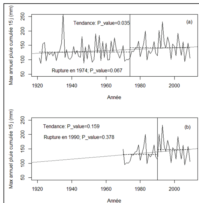
Figure 7 : Analyse de tendance et de rupture de la série des maxima annuels des pluies cumulées sur 15 jours pour la période 1920-2010 (a) et 1970-2010 (b). Trend/rupture analysis of the maximum annual cumulative rainfall over 15 days for the (a) 1920-2010 and (b) 1970-2010 periods.
